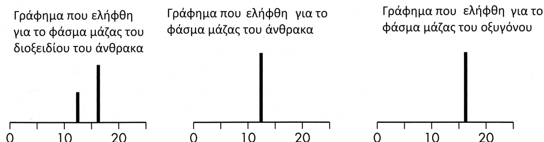
Σχήμα 5. Τα φάσματα μάζας της ένωσης διοξείδιο του άνθρακα και των συστατικών στοιχείων της άνθρακα και οξυγόνου.
