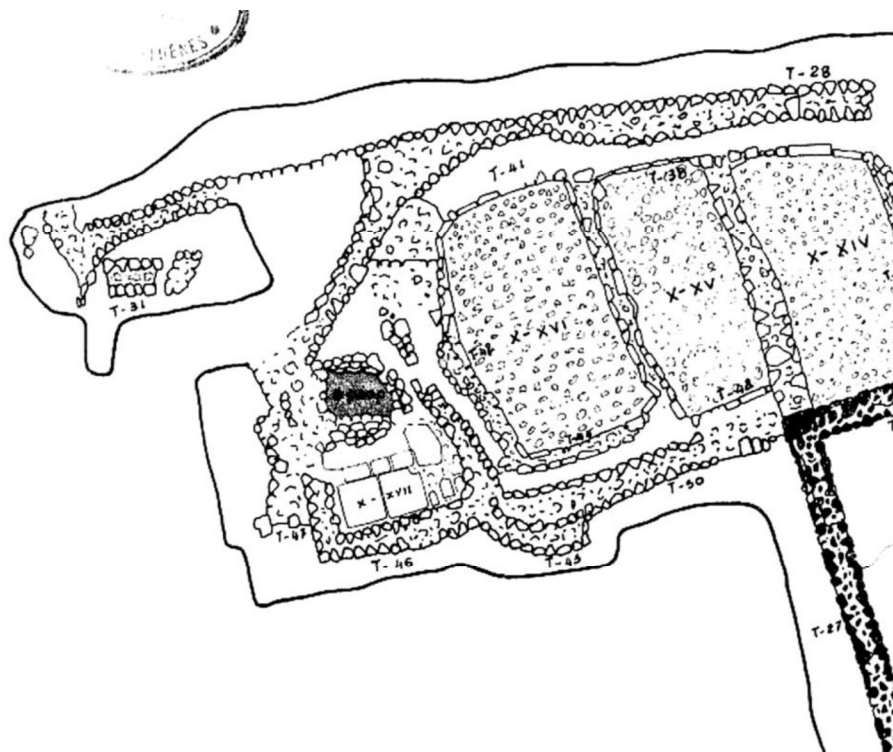
Εικ. 18: Βασιλική της Άφωτης Καρπάθου. Αποτύπωση των δεξαμενών (Κόλλιας, Άνασκαφή εις Άφωτην Καρπάθου», παρενθ. πιν. Η΄).
